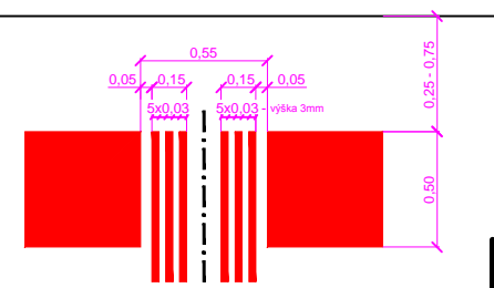
VZOR PROVEDENÍ DETAILU PŘECHODU PRO CHODCE S VODÍM PÁSEM PŘECHODU PRO SLABOZRACÉ
