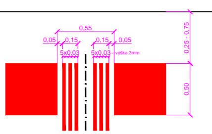
VZOR PROVEDENÍ DETAILU PŘECHODU PRO CHODCE S VODIČÍM PÁSEM PŘECHODU PRO SLABOZRAKÉ
