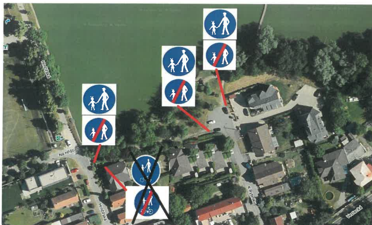
Situace návrhu osazení svislého dopravního značení C7a a C7b.
