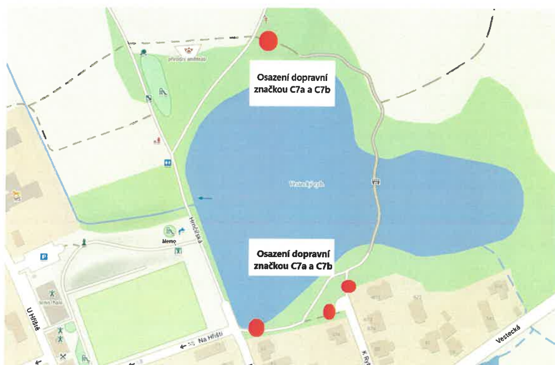
Celková situace návrhu osazení svislého dopravního značení C7a a C7b.
