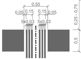
VZOR PROVEDENÍ DETAILU PŘECHODU PRO CHODCE S VODÍCÍM PÁSEM PŘECHODU PRO SLABOZRAKÉ
