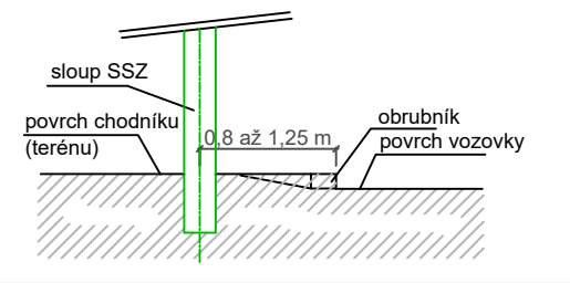
VZOR OSAZENÍ SLOUPŮ SSZ OD HRANY VOZOVKY
