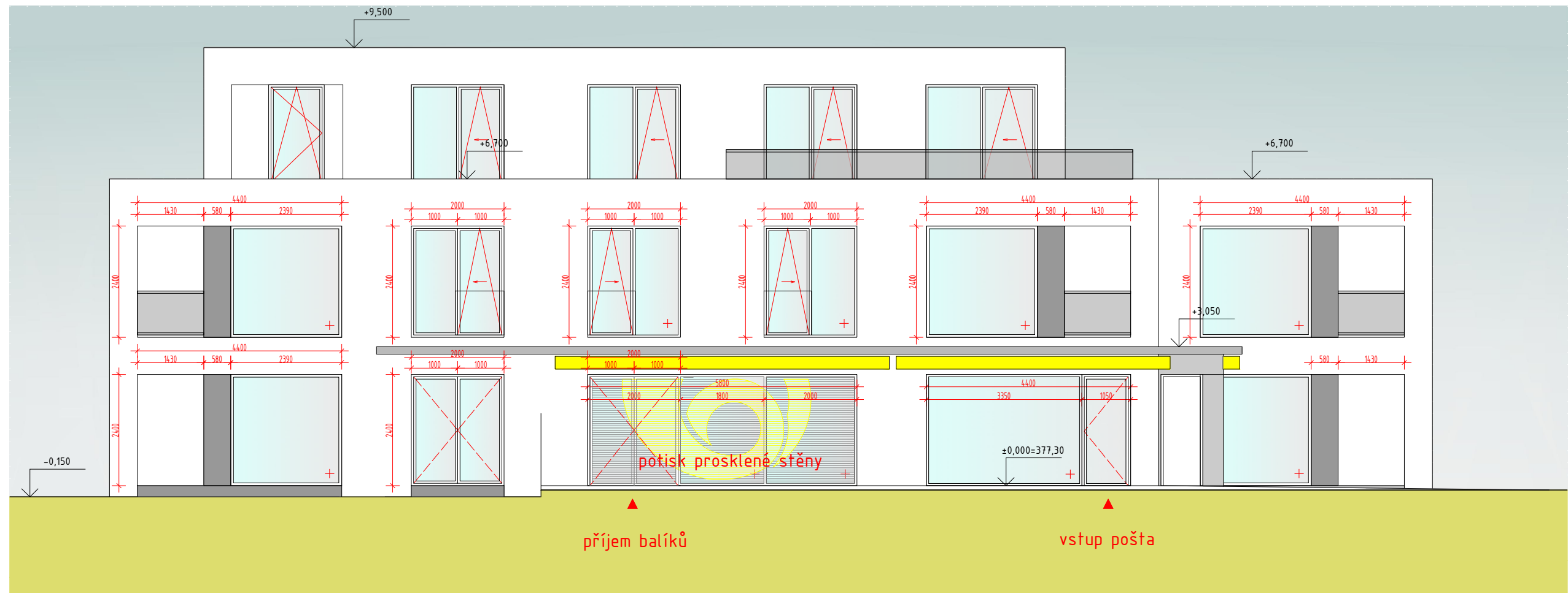
pohled západní
